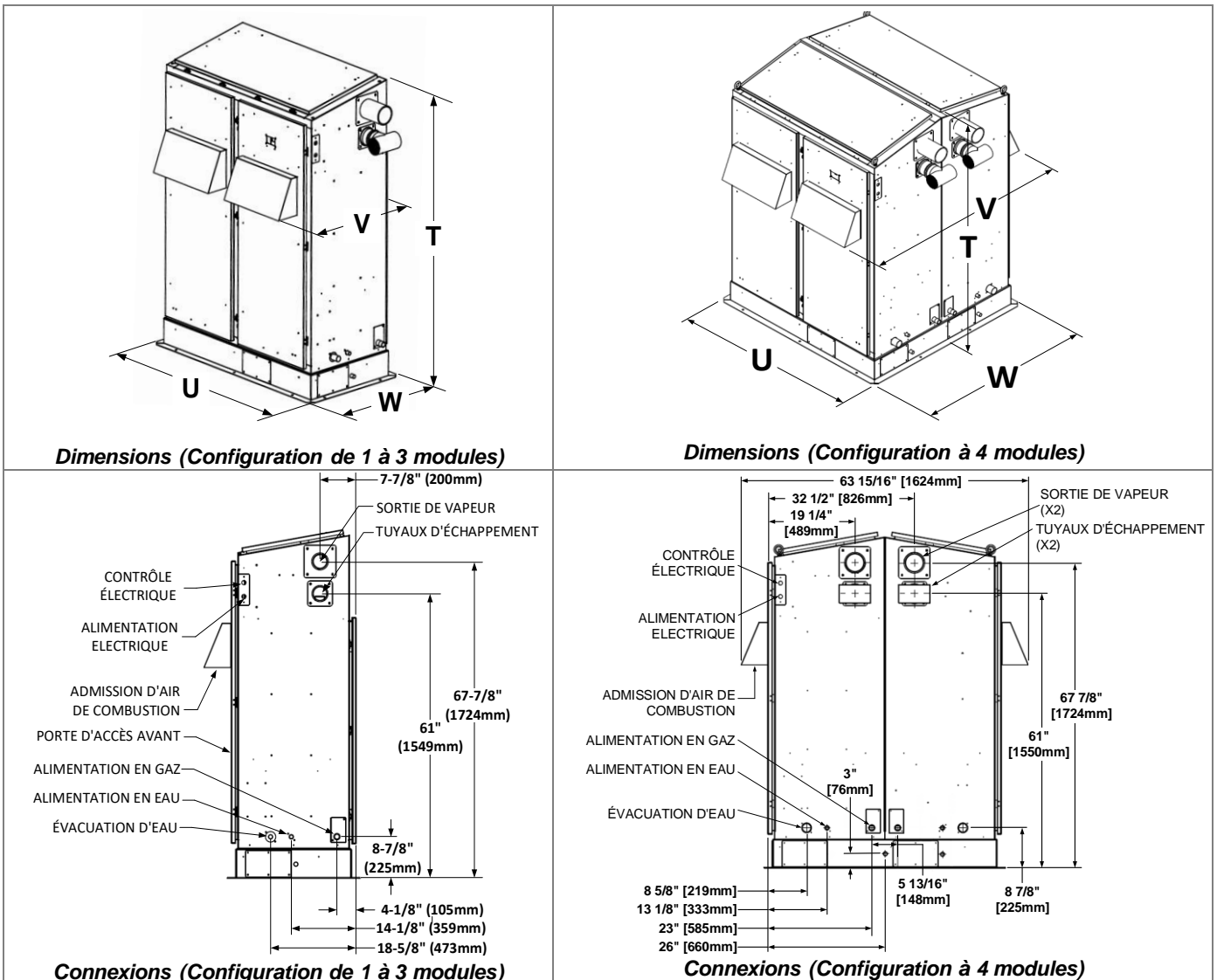
Illustration 6 - Boîtier extérieur
