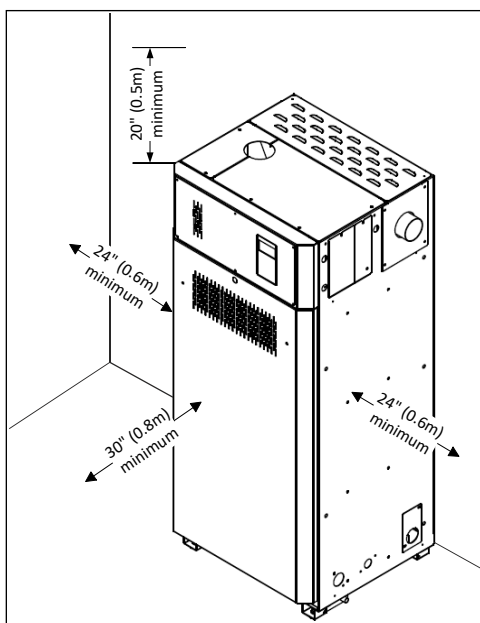
Illustration 9 - Dégagements pour humidificateur standard
