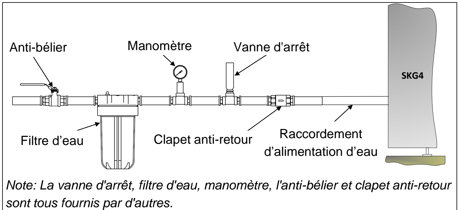
Illustration 28 - Connexion d'alimentation d'eau
